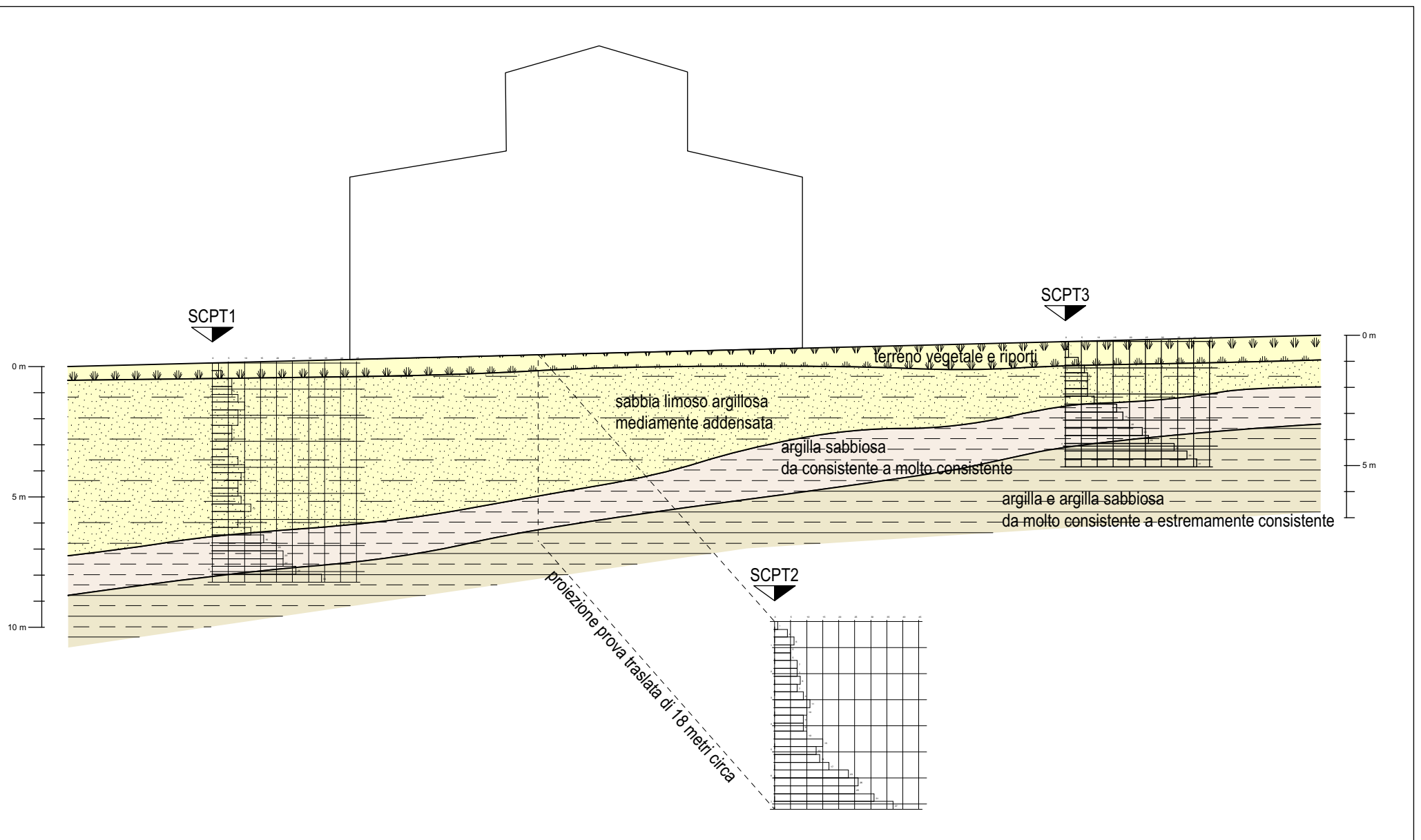
Figura 9 - SEZIONE LITOSTRATIGRAFICA INTERPRETATIVA
